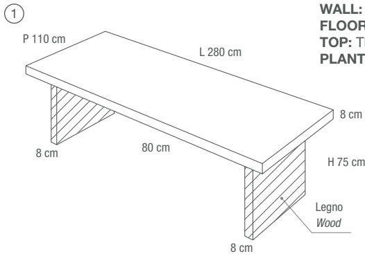
TAVOLO “HEAVY” LAVORAZIONE A “DOPPIA ELLE” CON GAMBE SMONTABILI IN LEGNO LISTELLARE, IMPIALLACCIATO ROVERE
