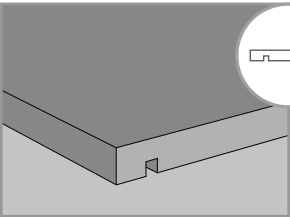
“SCANALATURA ROMPIGOCCIA” DRIP GROOVE FOR SILL
